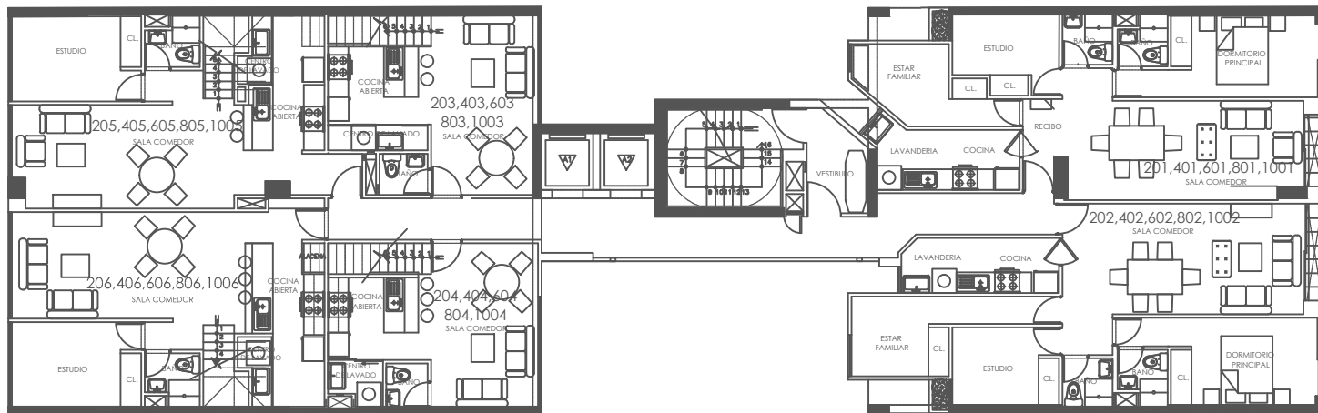
PISO TIPICO 2°,4°,6°,8° y 10° PISO 1/200
